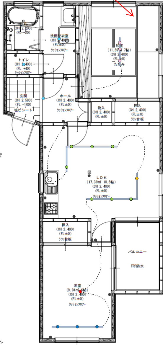
【床】 LDK柱部のコンセントは鋼製配管
